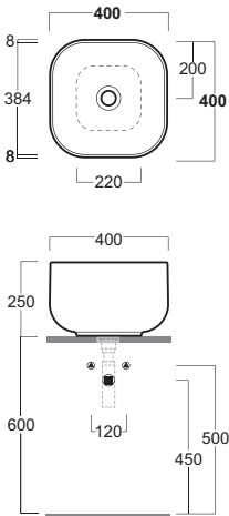
BA 04 Lavabo quadrato alto d'appoggio Square countertop washbasin with high rim 40.40.h25
