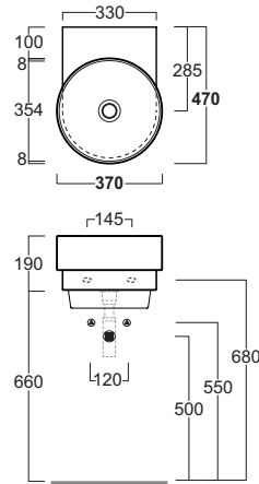
PO 05 Lavabo tondo da appoggio o sospeso Round washbasin wall hung or counter top Ø37.43.h19
