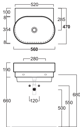
PO 06 Lavabo ovale da appoggio o sospeso Oval washbasin wall hung or counter top 56.43.h19
