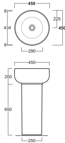
CN 301 Colonna rotonda per BA 01 per installazione centro stanza Rounded pedestal for BA 01 for center room installation 27,5.h65
