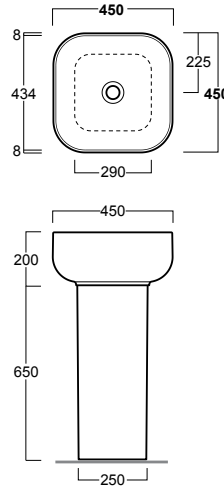
CN 401 Colonna quadrata per BA 03 per installazione centro stanza Squared pedestal for BA 03 for center room installation 27,5.h65
