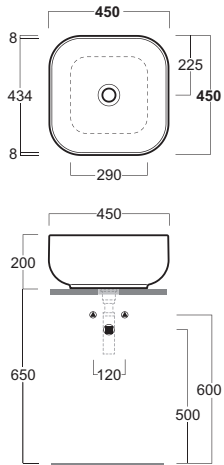
BA 03 Lavabo quadrato d'appoggio Square countertop washbasin 45.45.h20
