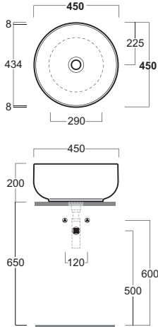
BA 01 Lavabo tondo d'appoggio Round countertop washbasin Ø45.h20
